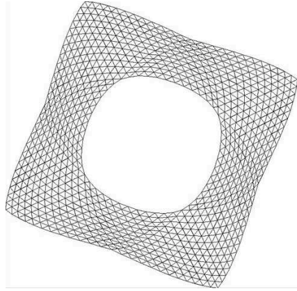
(d) Jagmesh1; |V| = 936, |E| = 2664 .
