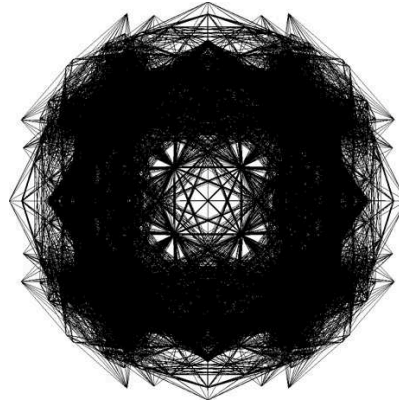
(d) Vibrobox; |V| = 12328, |E| = 165250 .
