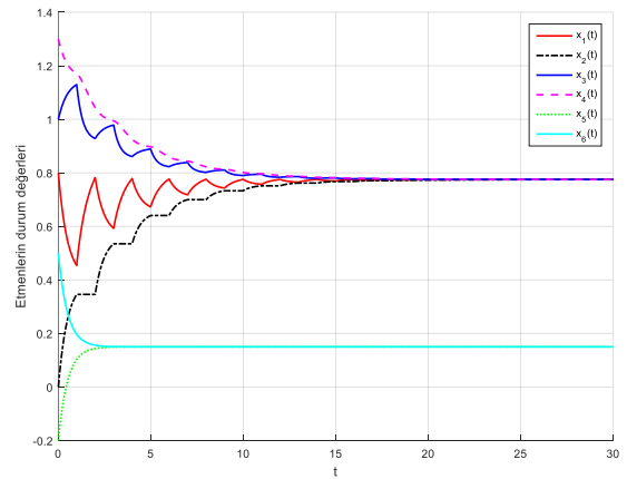
Şekil 4. (a) ve (b) ilingeleri arasında değişen ağın onaylaşımı.
